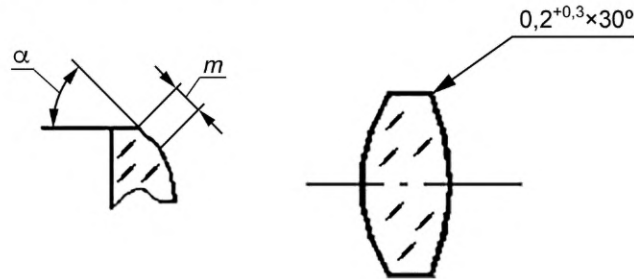
Рисунок 4 — Пример изображения фасок на чертеже
