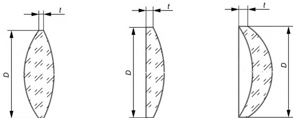
Рисунок 3 — Минимально допустимая толщина положительных линз
