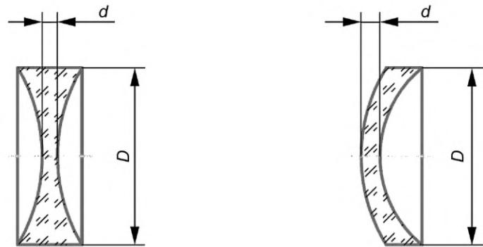
Рисунок 2 — Минимально допустимая толщина линзы по оси
