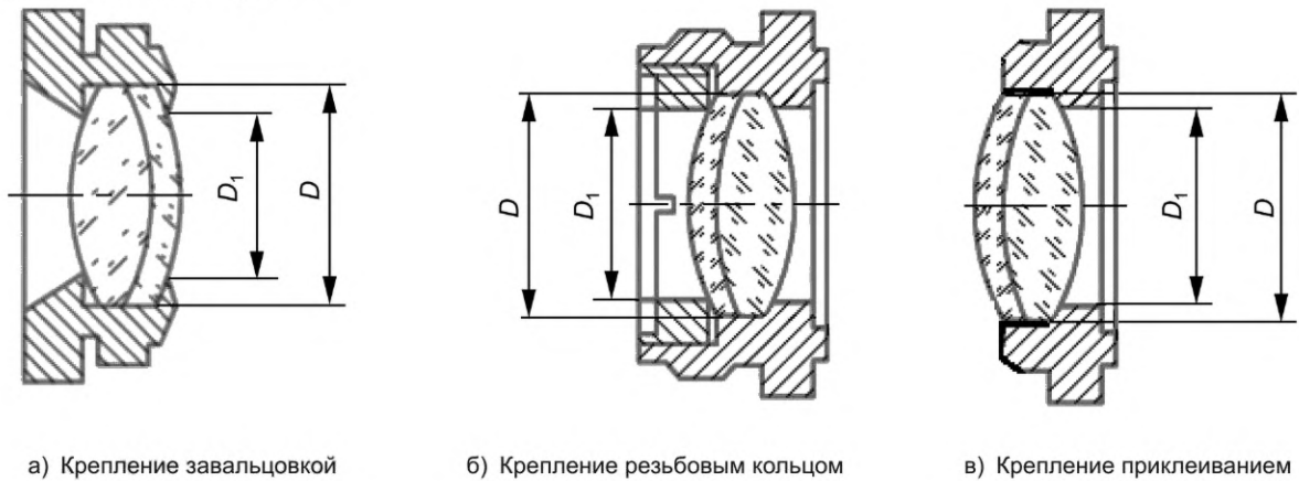
Рисунок 1 — Виды крепления
