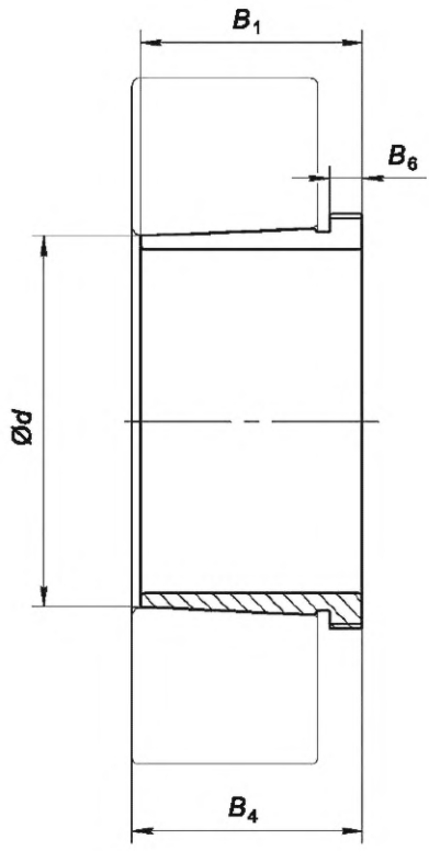
Рисунок 5 — Стяжная втулка
