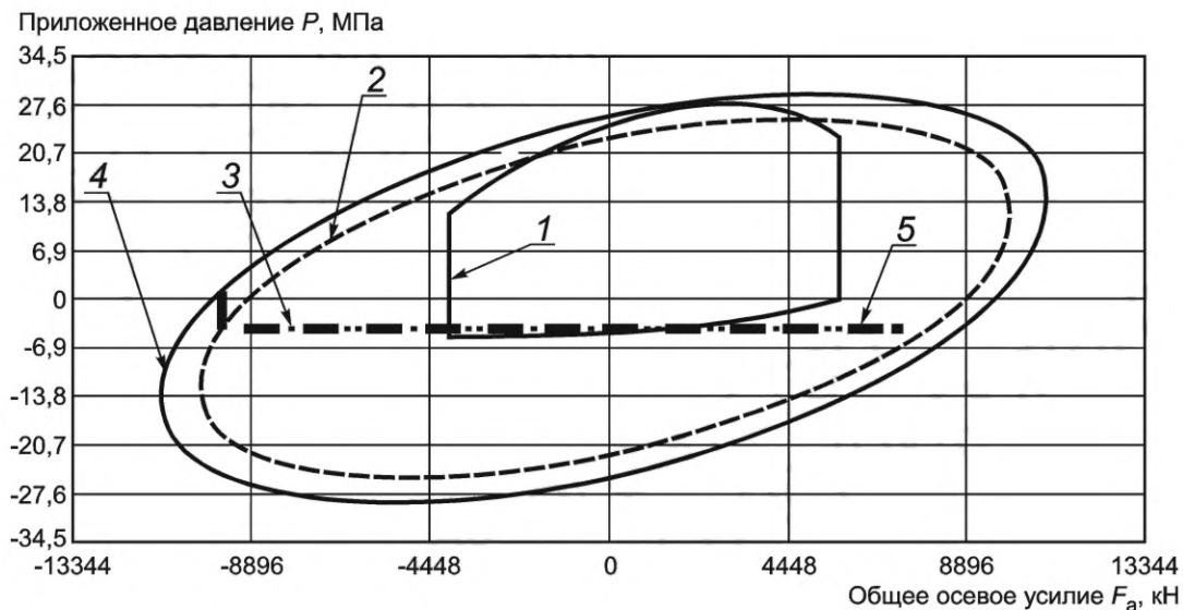
Рисунок D.39 — СЕЕ а испытательного образца
