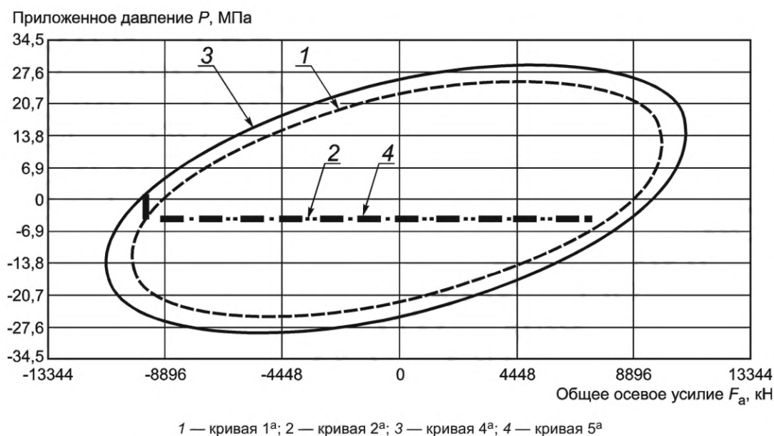
Рисунок D.38 — Эталонные характеристики испытательного образца тела трубы (кривые 1 a , 2 a , 4 a и 5 a )
