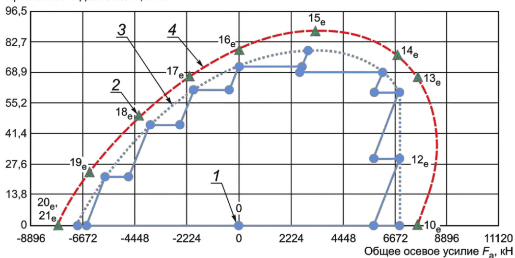
Рисунок D.28 — A e 90 % (QIII, QIV) и A e 90 % (QIV, QIII), TS-A этапы нагрузки 52—74
