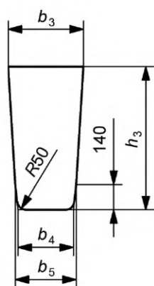
1 — испытательный шаблон в пространстве между стойками брусьев
