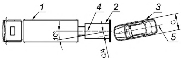
б — схема № 2: наезд в торцевую плоскость МФО со смещением на C/4 относительно оси МФО под углом 10°
