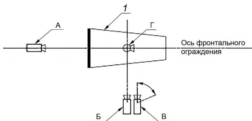
Рисунок 6 — Схема расположения видеокамер на испытательной площадке для испытаний ФО (вид сверху)
