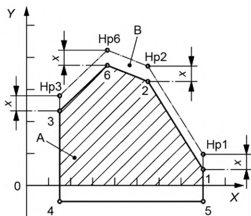
Рисунок 1 — Испытательная и рабочая диаграммы для одноступенчатых горелок (заштрихованная область — рабочая диаграмма)
