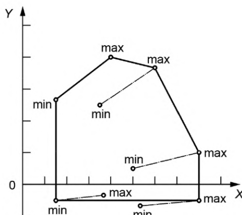
Рисунок 1 — Испытательная и рабочая диаграммы для одноступенчатых горелок (заштрихованная область — рабочая диаграмма)
