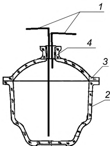
Рисунок А.1 — Стеклоная емкость (эксикатор), имеющая две отводные трубки, используемая для приготовления воздушной вытяжки
