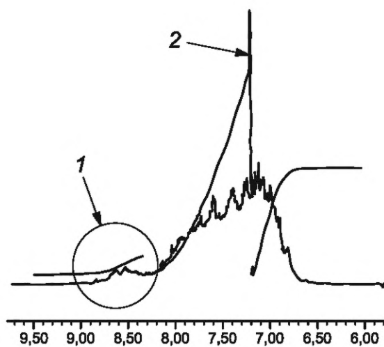
1 — область залива (8,3—9,5 ppm); 2 — примесь \text{CHCl}_3
