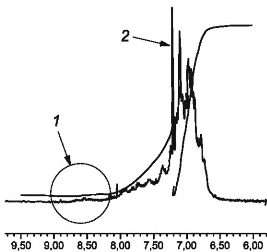
1 — область залива (8,3—9,5 ppm); 2 — примесь \text{CHCl}_3
