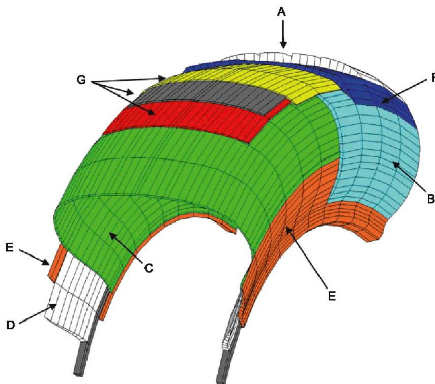
Рисунок В.1 — Конструкция покрышки
