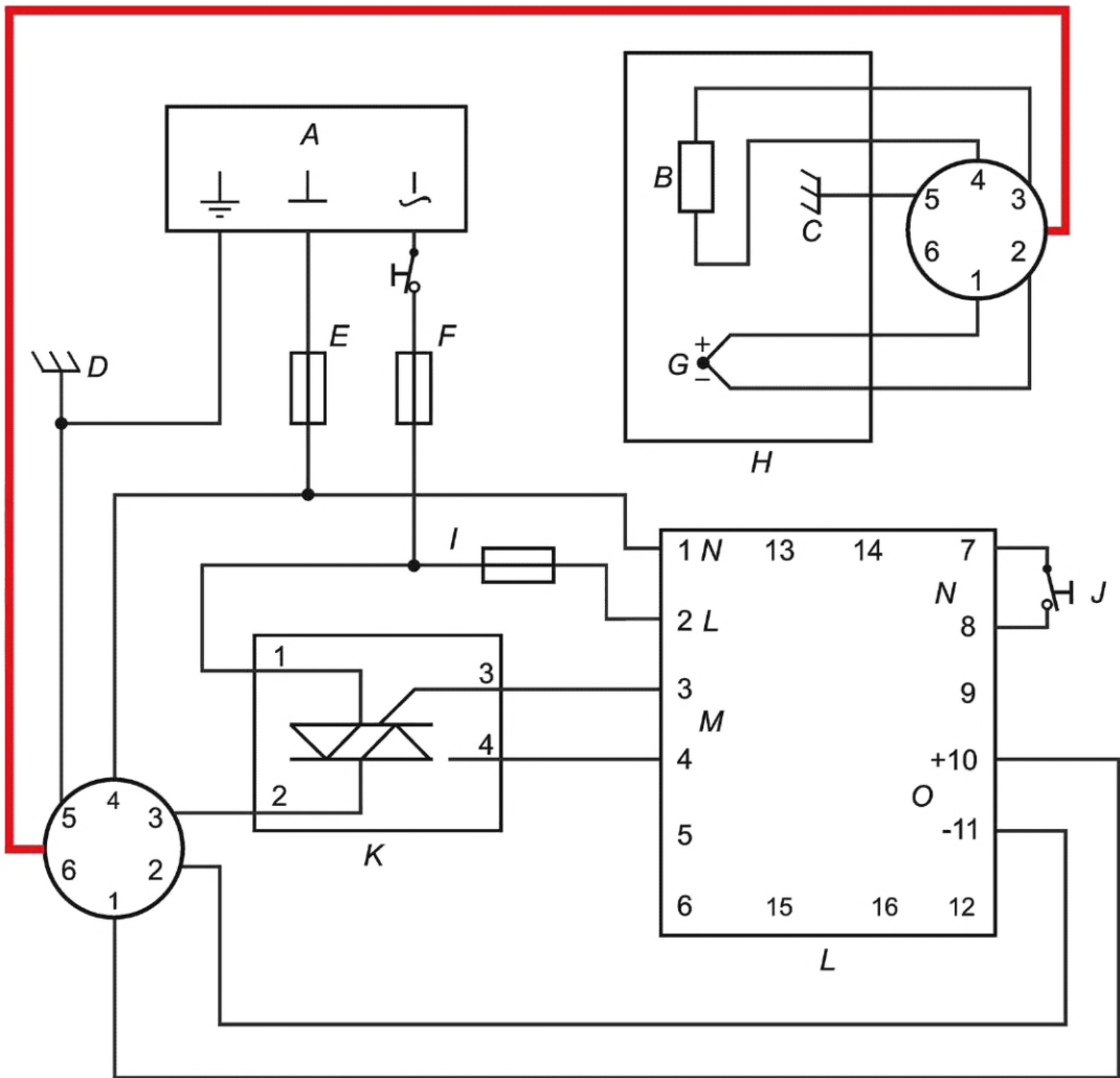
A — питание от сети 230 В переменного тока; B — нагревательный провод; C — заземление; D — заземлительная коробка; E — предохранитель F630 мА; F — предохранитель F630 мА; G — термopара типа К (NiCrNi); H — нагревательный картридж HotSet HotRod 8×80 200 Вт; I — предохранитель 200 мА; J — пусковой переключатель; K — твердотельное реле croud D2425; L — терморегулятор HotSet HotControl C248; M — doul2; N — цифровой вход; O — термомолния
