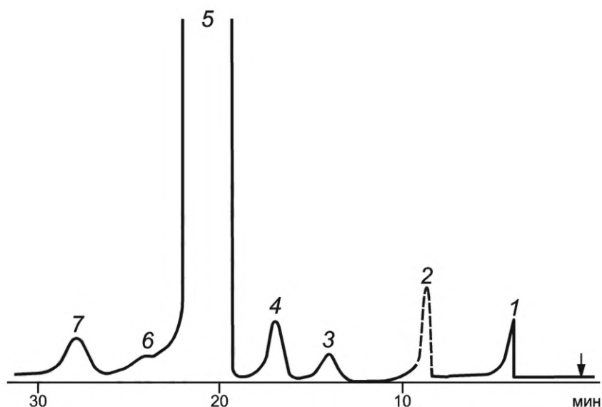
Рисунок 2 — Типовая хроматограмма о-крезола
