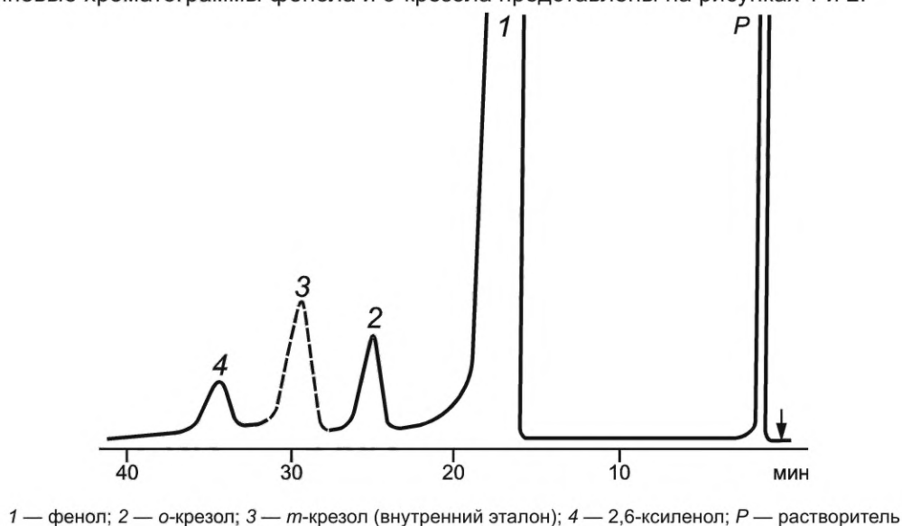
Рисунок 1 — Типовая хроматограмма фенола
