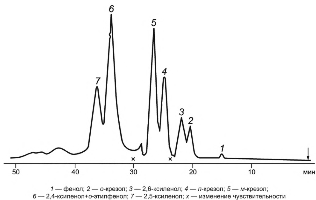
Рисунок 1 — Типовая хроматограмма дикрезолола
