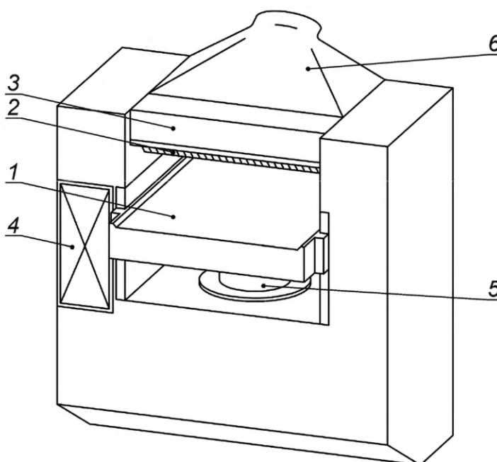
1 — загрузочный стол; 2 — устройство, предотвращающее обратный удар; 3 — верхнее защитное ограждение; 4 — панель управления; 5 — механизм вертикального перемещения стола; 6 — вытяжной колпак
