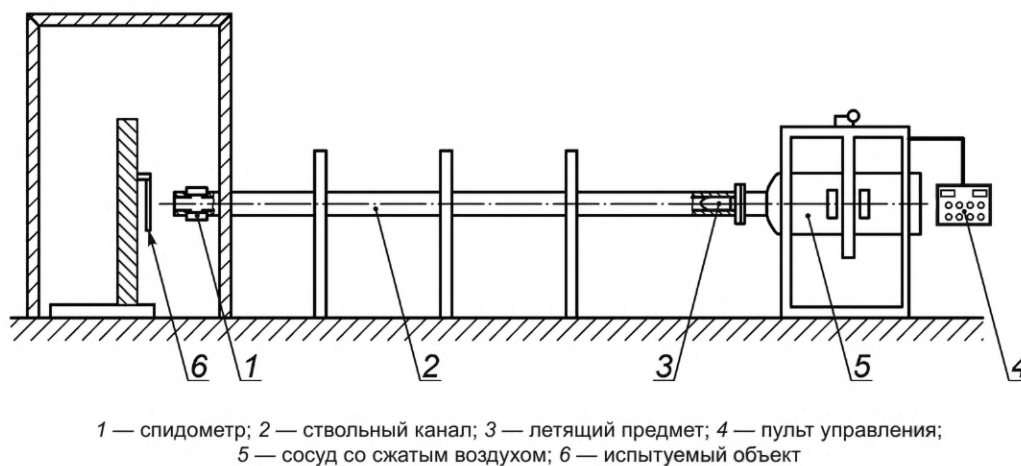
Рисунок С.1 — Пример оборудования для проведения испытаний на удар
