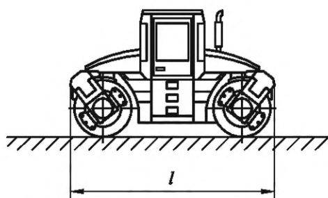
а) Двухвальный дорожный каток
