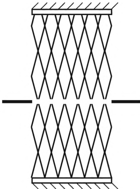
Рисунок 1 — Схема закрепления образца в разрывной машине
