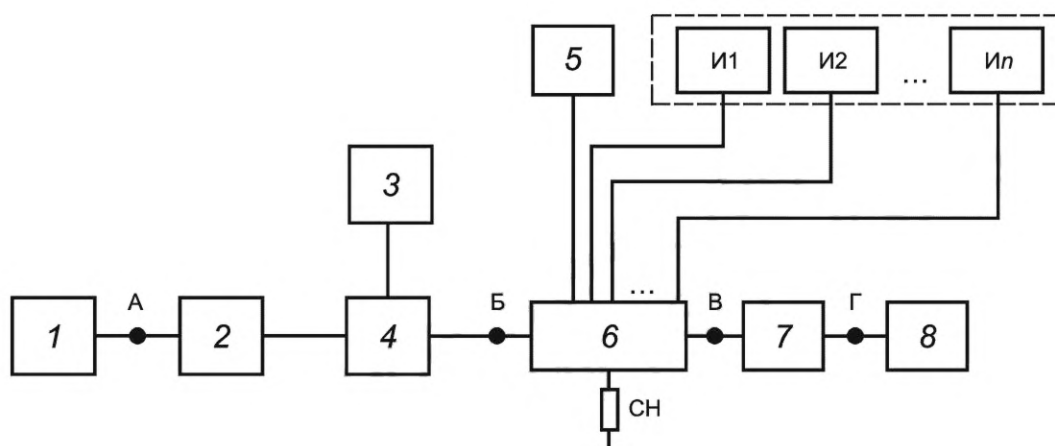
1 — СВЧ-генератор; 2 — изолятор; 3 — измеритель мощности; 4 — направленный ответвитель; 5 — источник питания; 6 — ИУ; 7 — аттенюатор; 8 — анализатор спектра; И1, И2... Ип — источники управления
