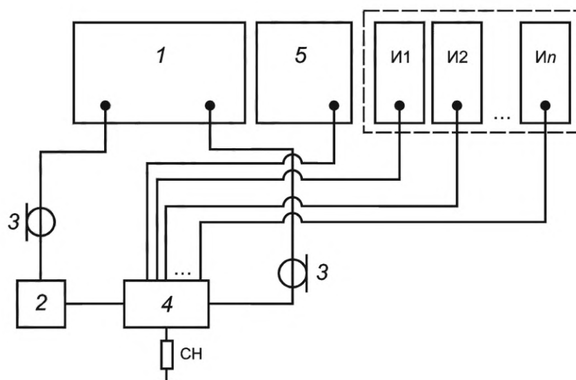
1 — ВАЦ; 2 — СВЧ-предусилитель; 3 — СВЧ кабельные сборки; 4 — ИУ; 5 — источник питания; И1, И2... Ил — источники управления; СН — согласованная нагрузка
