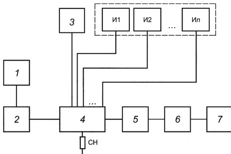
1 — СВЧ-генератор; 2 — СВЧ-предусилитель; 3 — источник питания; 4 — ИУ; 5 — полосно-пропускающий фильтр; 6 — аттенюатор; 7 — детектор СВЧ-мощности; И1, И2... И n — источники управления; СН — согласованная нагрузка
