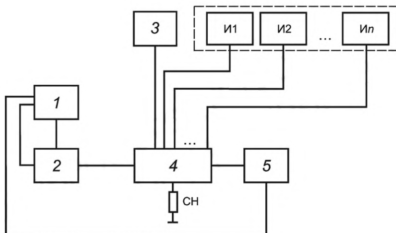
1 — скалярный анализатор цепей; 2 — датчик КСВН; 3 — источник питания; 4 — ИУ; 5 — детекторная головка; И1, И2... Ип — источники управления; СН — согласованная нагрузка
