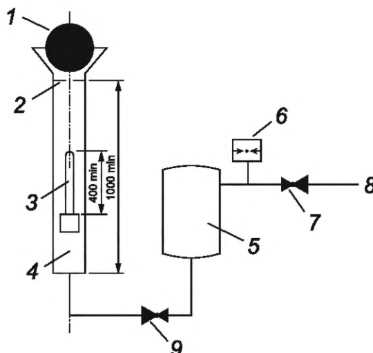
1 — мяч; 2 — упор; 3 — боек; 4 — направляющая труба; 5 — емкость со сжатым воздухом; 6 — манометр; 7 — редуцирующий проходной клапан; 8 — воздухопровод от компрессора; 9 — клапан
