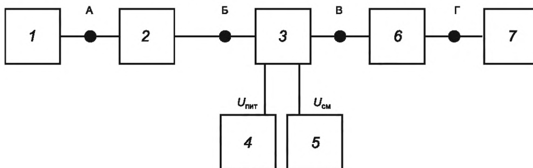
1 — СВЧ-генератор; 2 — изолятор; 3 — ИУ; 4 — источник питания; 5 — источник напряжения смещения; 6 — аттенуатор; 7 — АС; U_{\text{пит}} и U_{\text{см}} — напряжения питания и смещения соответственно
