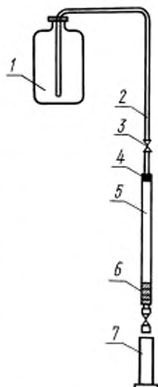
1 — бутылка вместимостью 10—20 дм 3 ; 2 — сифон; 3 — зажим; 4 — пробка; 5 — цилиндрическая стеклянная трубка (диаметр — 16,5±0,5 мм; h ≥ 850 мм); 6 — фильтр (пористая стеклянная пластинка); 7 — цилиндр
