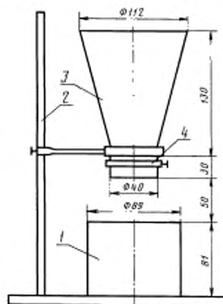
Прибор для определения насыпной плотности
