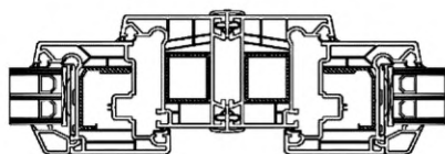
а) Торцевое соединение коробок с использованием мини-соединителей
