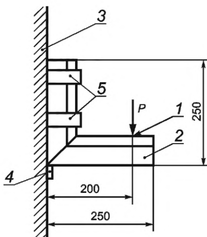
1 — точка приложения нагрузки; 2 — испытательный образец; 3 — вертикальная опора; 4 — упор; 5 — хомуты для крепления образца; P — поперечная нагрузка, действующая на угловое соединение
