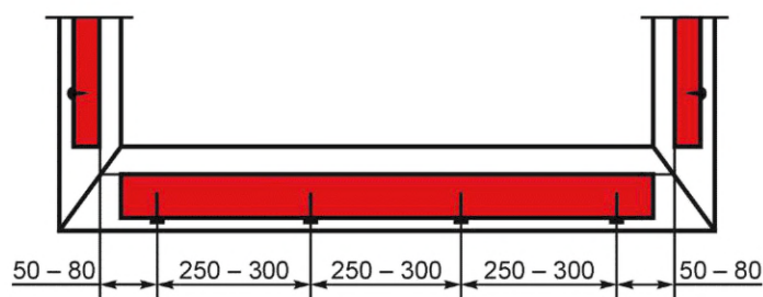
а) Схема крепления усилительных вкладышей в профилях ПВХ белого цвета
