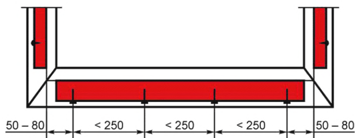
б) Схема крепления усилительных вкладышей в цветных профилях ПВХ
