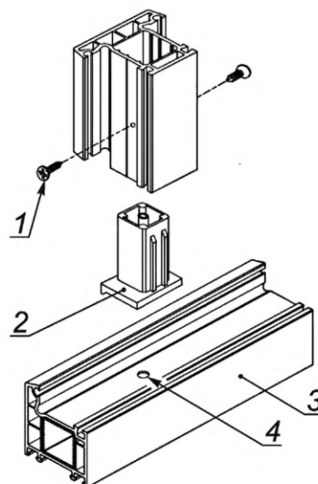
1 — шурупы; 2 — соединитель импоста; 3 — рама; 4 — отверстие
