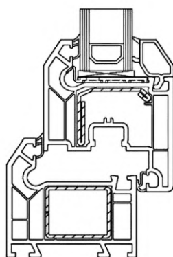
б) Оконный блок из четырехкамерных профилей
