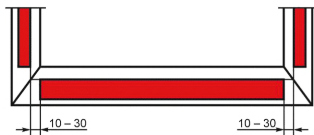
Рисунок 9 — Пример установки усилительных вкладышей в профилях ПВХ
