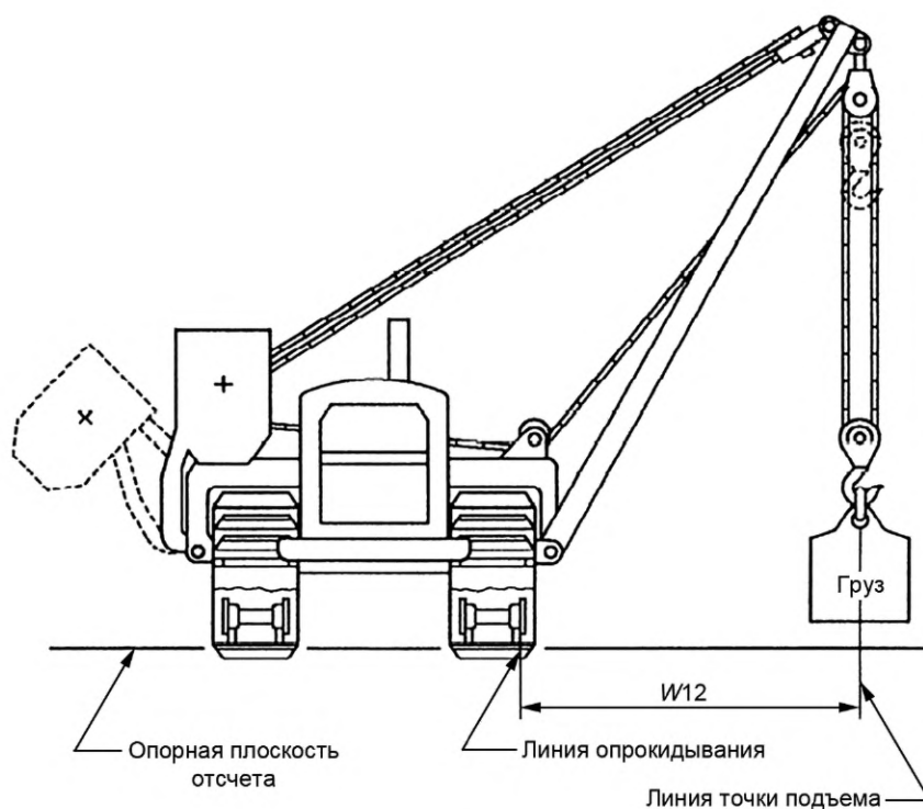
Рисунок 1 — Трубоукладчик
