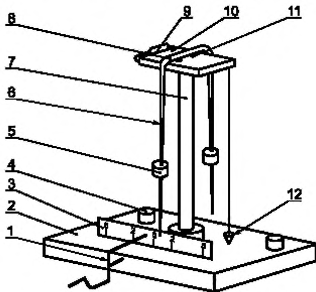
1 — пусковой механизм; 2 — основание; 3 — шкала; 4 — установочные винты; 5 — груз; 6 — двусторонний механизм; 7 — штатив; 8 — соединительная планка; 9 — рамка; 10 — столик; 11 — стальные шарики; 12 — отвес
