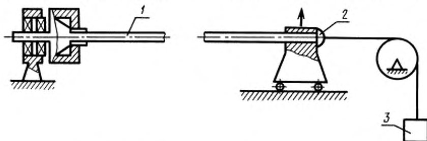
1 — броня; 2 — каретка с зажимом; 3 — груз для растяжения
