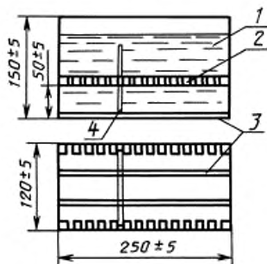
1 — жидкость; 2 — держатель образцов; 3 — рейки, на которых устанавливают образцы; 4 — образец
