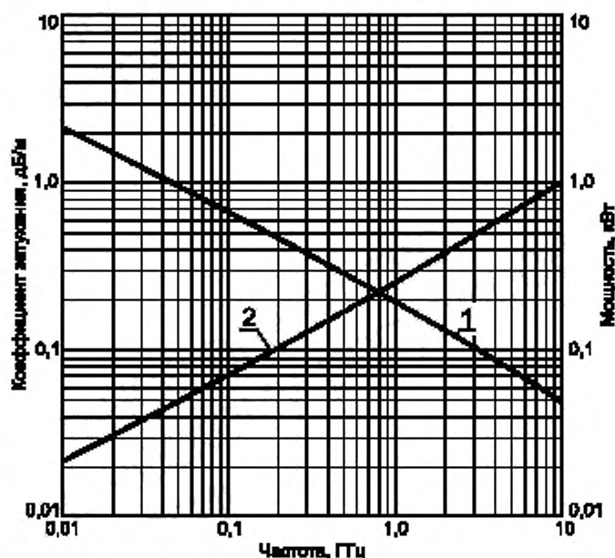
Частотные зависимости
