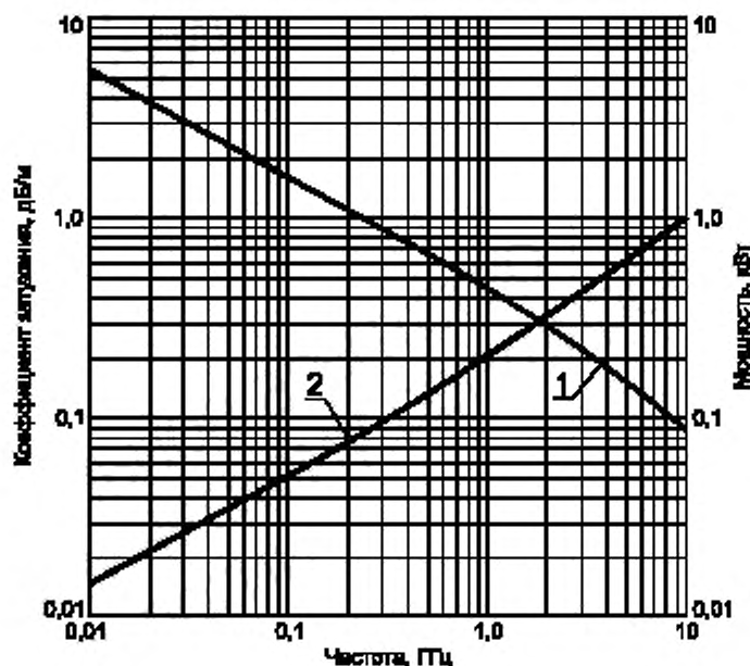
Частотные зависимости
