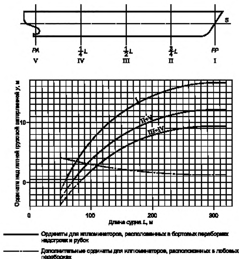
Рисунок В.2 — Графики определения ординат расположения прямоугольных иллюминаторов типа Е для мест, указанных в 3.2, кроме кормовых концевых переборок
