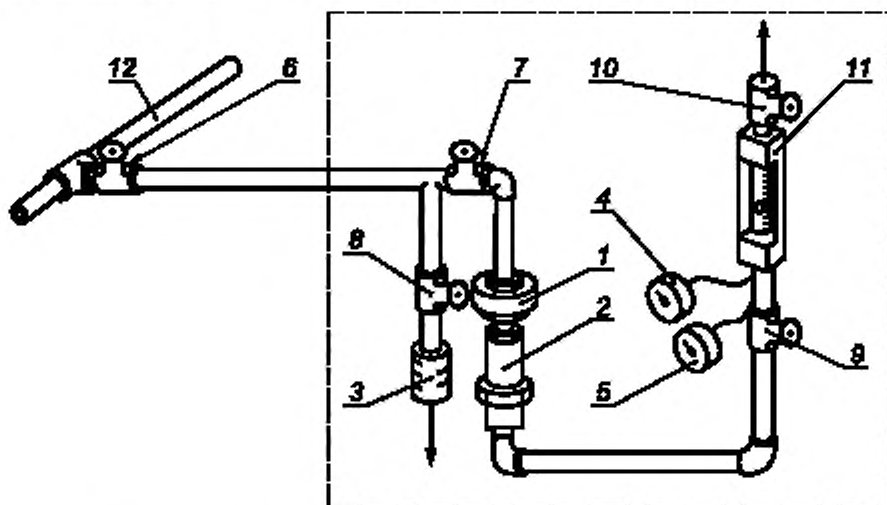
1 — патрон мембраны а) ; 2 — трубка из нержавеющей стали (см. рисунок А.2) для сбора паров масла и органических растворителей; 3 — глушитель; 4 — манометр; 5 — термометр; 6—8 — запорные клапаны; 9 — вентиль регулирования потока; 10 — вентиль регулирования потока б) ; 11 — расходомер; 12 — основная труба
