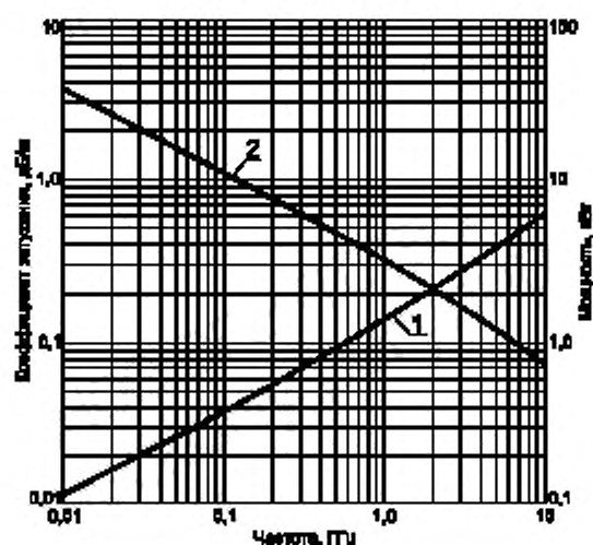
Частотные зависимости
