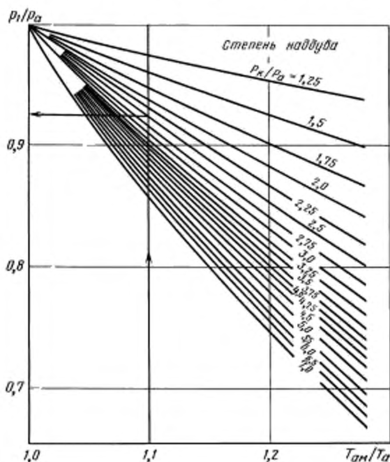
Диаграмма для определения давления на входе в компрессор при имитации высокой температуры воздуха в условиях на месте установки дизеля
