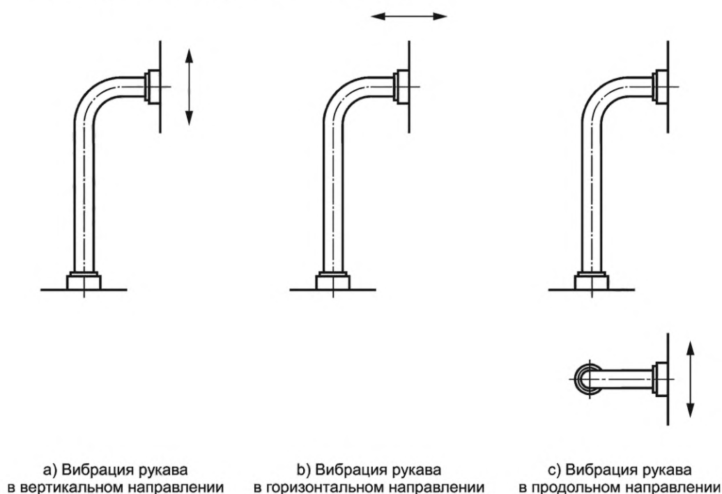
Рисунок С.1 — Направления вибрации испытываемого образца
