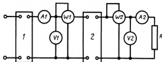
1 — регулятор напряжения; 2 — испытуемый трансформатор; R — номинальная нагрузка (резистор)
