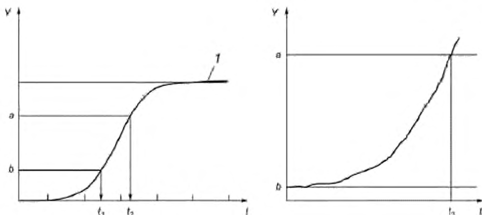
Y — скорость проникновения, \text{мкг} \cdot \text{см}^{-2} \cdot \text{мин}^{-1} ; t — время, T — проникновение при установившемся режиме; a — нормализованная скорость проникновения (NPR); b — минимально распознаваемая скорость проникновения; t_2 — нормализованное время проникновения (NBT)
