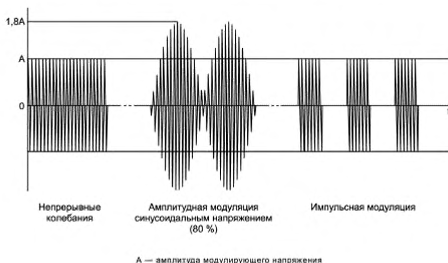
Рисунок 3 — Виды модуляции
