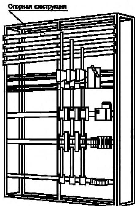
Рисунок С.1 — НСУ заводского изготовления открытого типа
