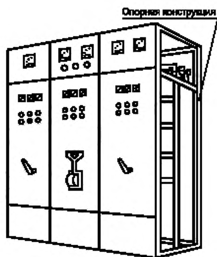
Рисунок С.2 — НСУ заводского изготовления открытого типа, защищенное спереди
