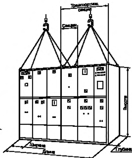
Рисунок С.4 — НКУ заводского изготовления много- шкафного типа
