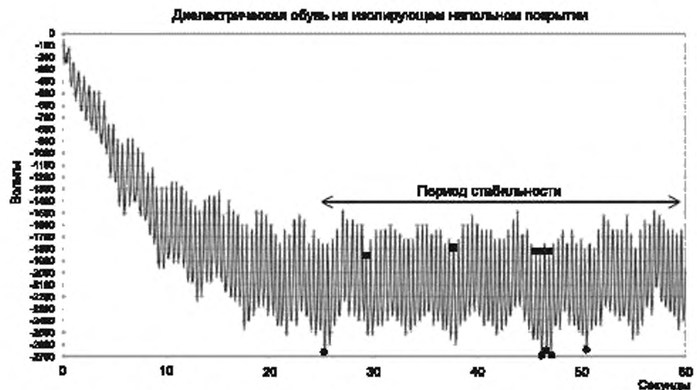
б) Осциллограмма напряжения человеческого тела отрицательной полярности
