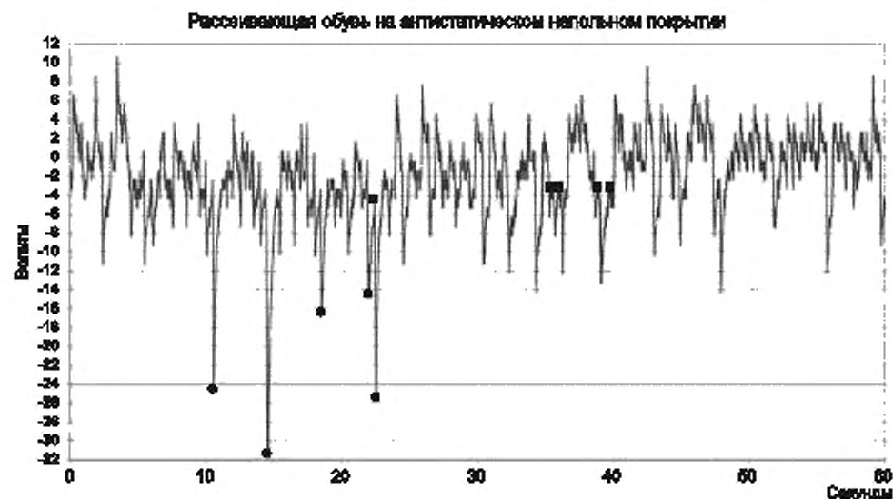
а) Осциллограмма напряжения человеческого тела с положительными и отрицательными точками
