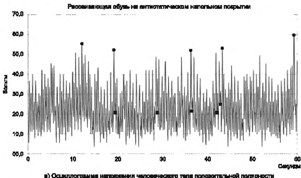
Рисунок 2, лист 1 — Типичные осциллограммы напряжения тела, показывающие пики, используемые для вычисления средних значений
