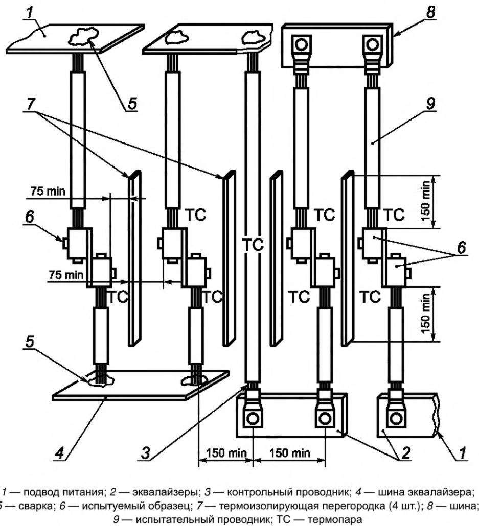
Рисунок L.1 — Испытательная установка
