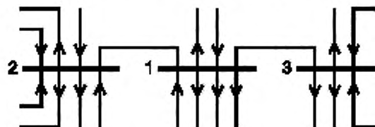
Рисунок 6 — Определение S_i для ячеистой системы ВН или СВН
