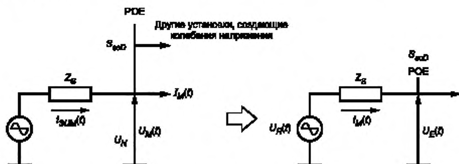
Рисунок Е.7 — Оценка уровня эмиссии с использованием текущих измерений
