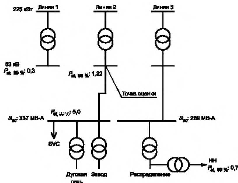
Рисунок G.6 — Конфигурация системы «л-1»
