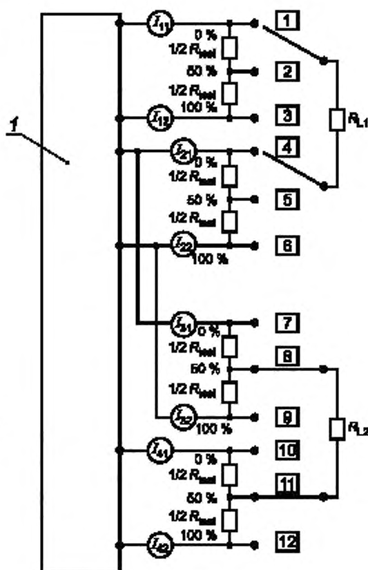
Рисунок F.4b — Электроды, соединенные параллельно
