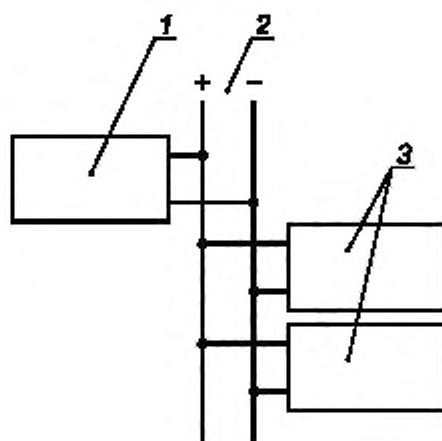
1 — управляющий прибор; 2 — ШИМ; 3 — регулируемый ЭПРА
