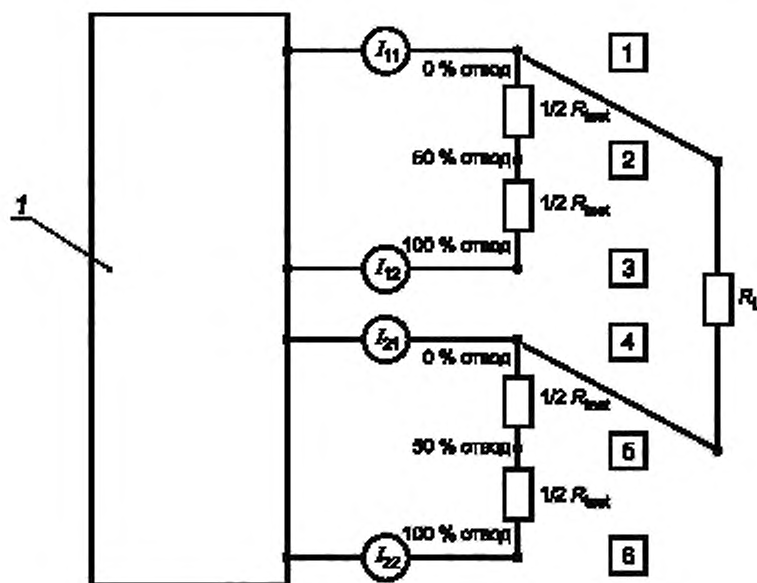
1 — испытательный ЭПРА, R_L — резистор, заменяющий лампу; I_{on} — измеряемый ток; 1...6 — положения переключателя
