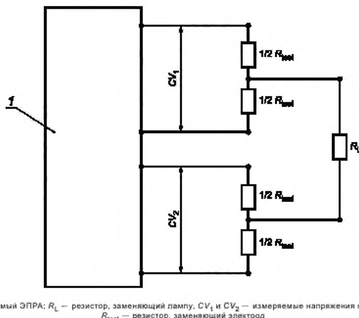
Рисунок 4 — Принципиальная схема установки для испытания на CV
