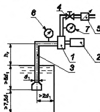
1 — насос, 2 — приводной двигатель; 3 — всасывающая линия; 4 — напорный вентиль, 5 — устройство для измерения подачи, 6, 7 — мановакуумметры; d_1 — условный диаметр всасывающих патрубков, h_r — геометрическая высота всасывания
