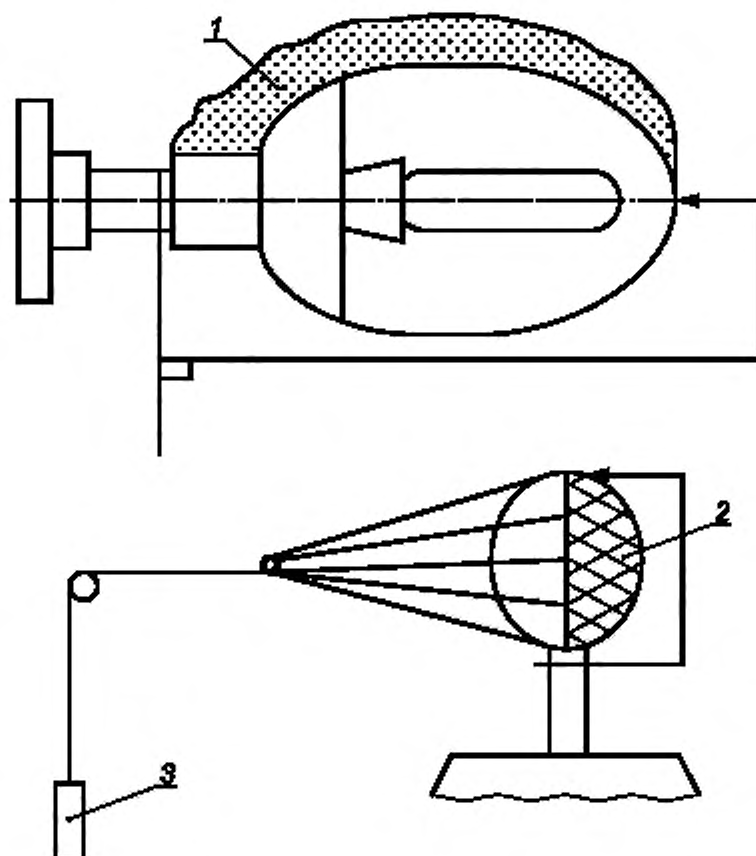
1 — мешок с песком; 2 — сетка; 3 — груз
