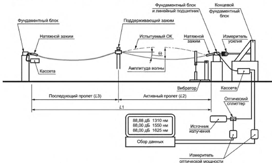
Рисунок 33 — Схема испытания ОК на галоирование (пояска ОК)
