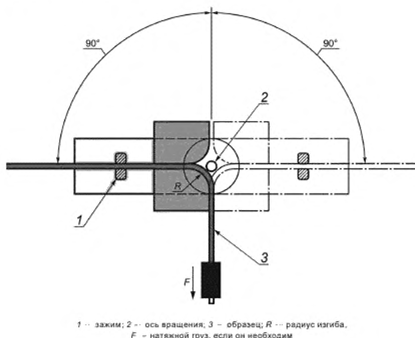
Рисунок 8 — Схема испытания на многократный изгиб ОК/кабельной сборки
