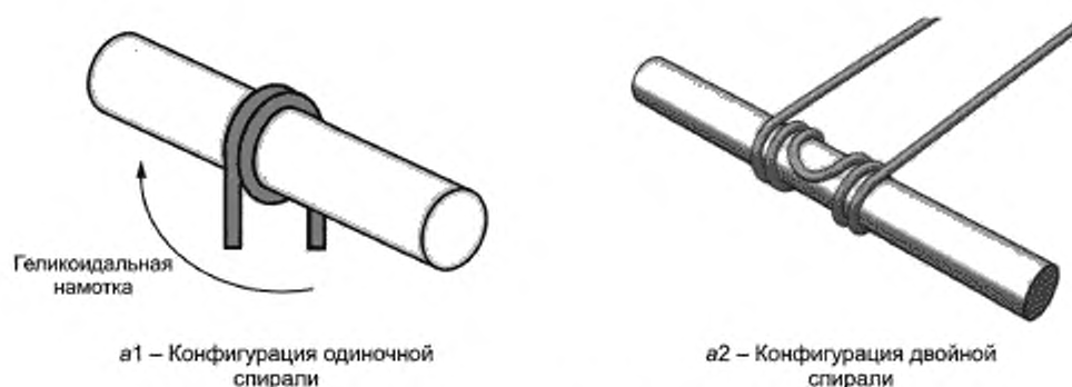
а — Схема оснастки для испытания по методу E11A
