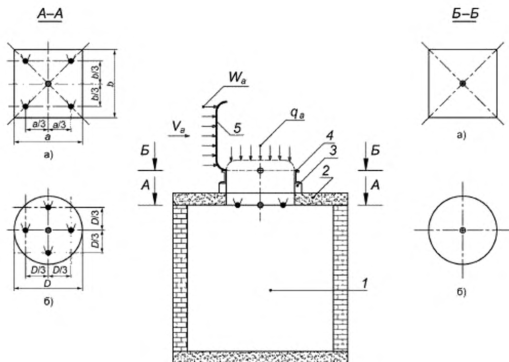
1 — печь с горелками; 2 — вкладыш покрытия печи; 3 — установочный элемент; 4 — корпус дымового люка; 5 — заслонка дымового люка; 6 — термозлемент привода; а) — дымовой люк прямоугольного сечения, б) — дымовой люк круглого сечения. Y — ТЭП; • — точка измерения статического давления; ⊕ — комбинированный приемник давления; V_a — скорость ветра (воздушного потока), W_a — ветровая нагрузка; q_a — механическая нагрузка
