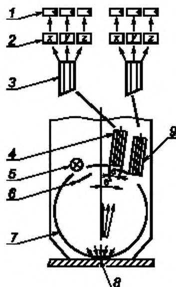
1 — фотодатчики, 2 — фильтры, 3 — световод, 4 — канал измерения, 5 — косвенная лампа-вспышка, 6 — затвор; 7 — фотометрический шар, 8 — образец под измерительной диафрагмой, 9 — опорный канал
