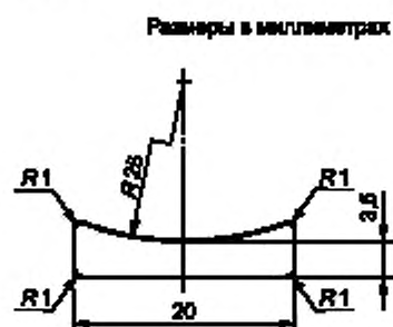
Рисунок 8 — Форма насадки для выдавливания выпечки
