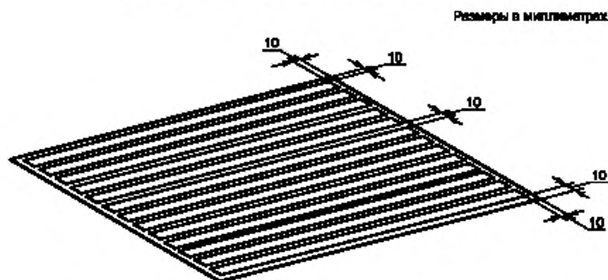
Рисунок 9 — Расположение полосок для выпечки на противне для выпекания
