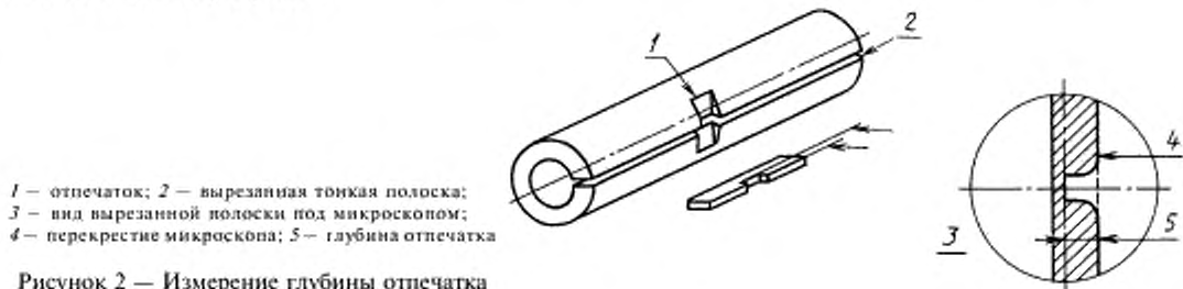
Рисунок 2 — Измерение глубины отпечатка
