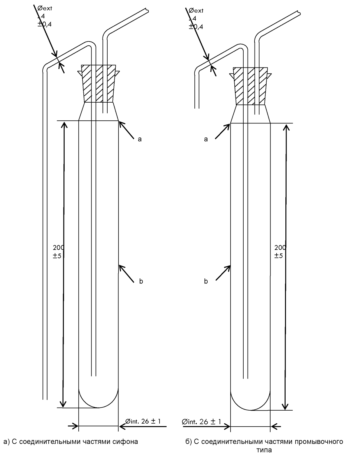
Рисунок В.1 — Примеры экстракционных пробирок
