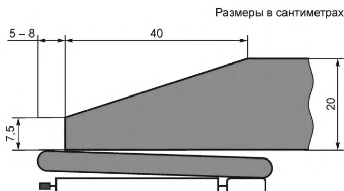
Рисунок 3 — Расположение матов
