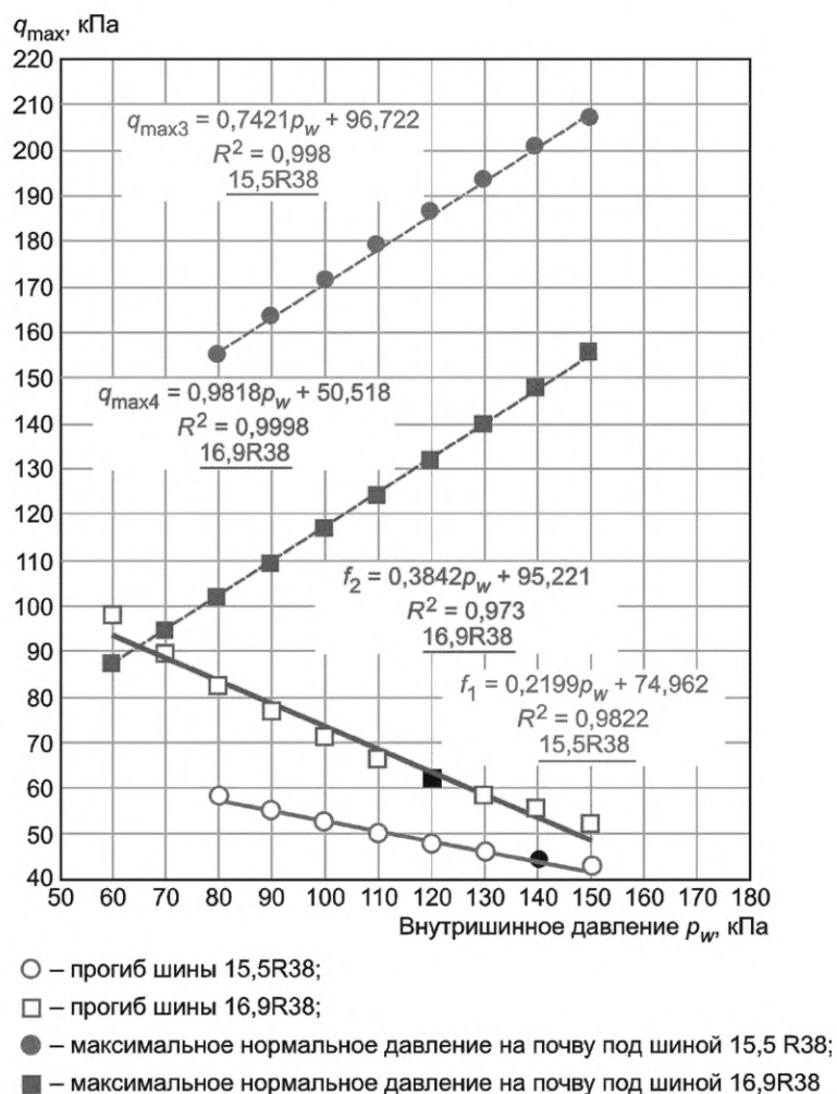
Рисунок В.3 — Зависимость изменения максимального нормального давления q_{\max}^k и нормального прогиба шины f от внутришинного давления p_w в шинах 15,5R38 и 16,9R38 при постоянной вертикальной нагрузке G_k = 15 кН
