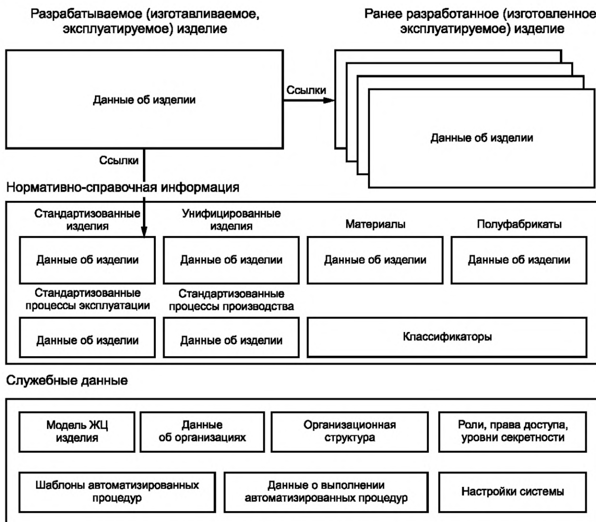
Рисунок 1 — Основные группы данных в АС УДИ
