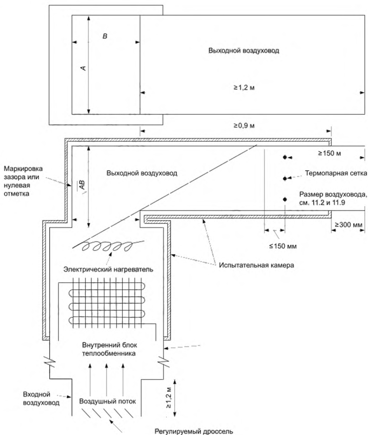
а) Схема для восходящего потока
