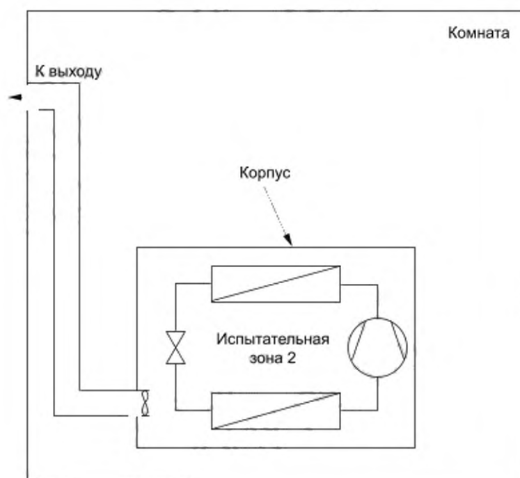
Рисунок GG.2 — Принудительная вентиляция
